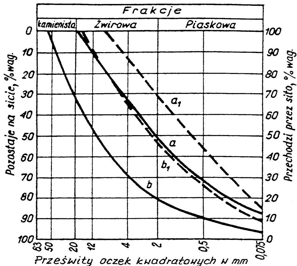
Rysunek 1. Obszar uziarnienia optymalnych mieszanek żwirowych
