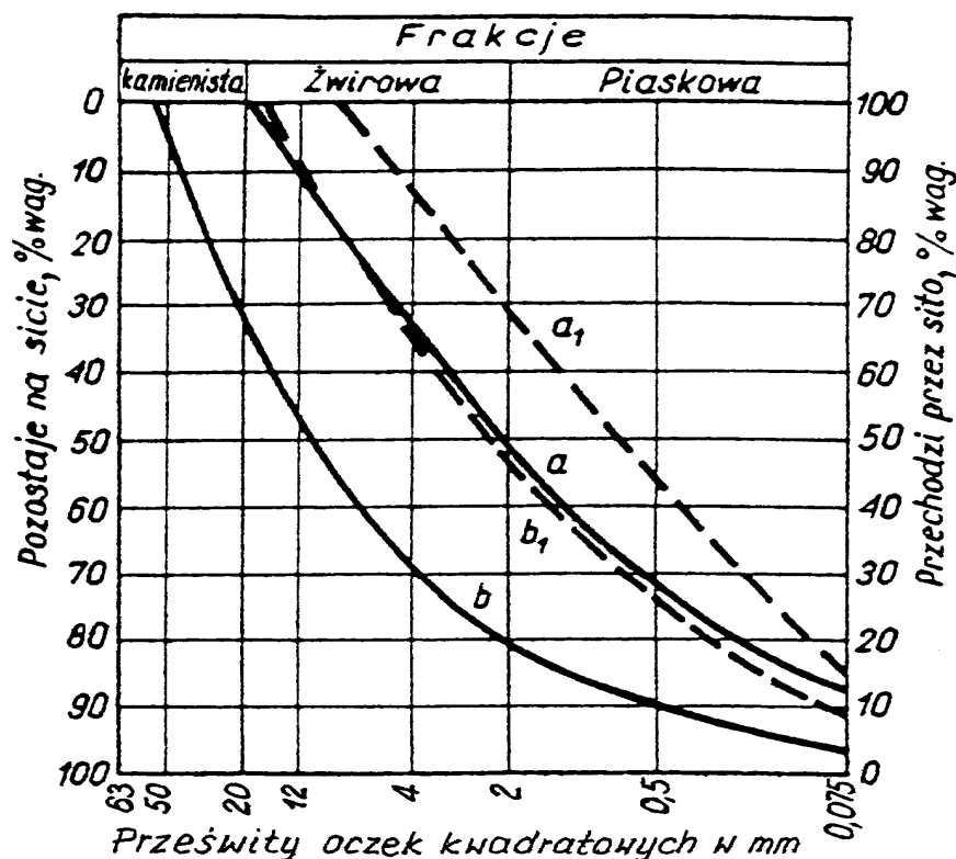
Rysunek 1. Obszar uziarnienia optymalnych mieszanki żwirowych
